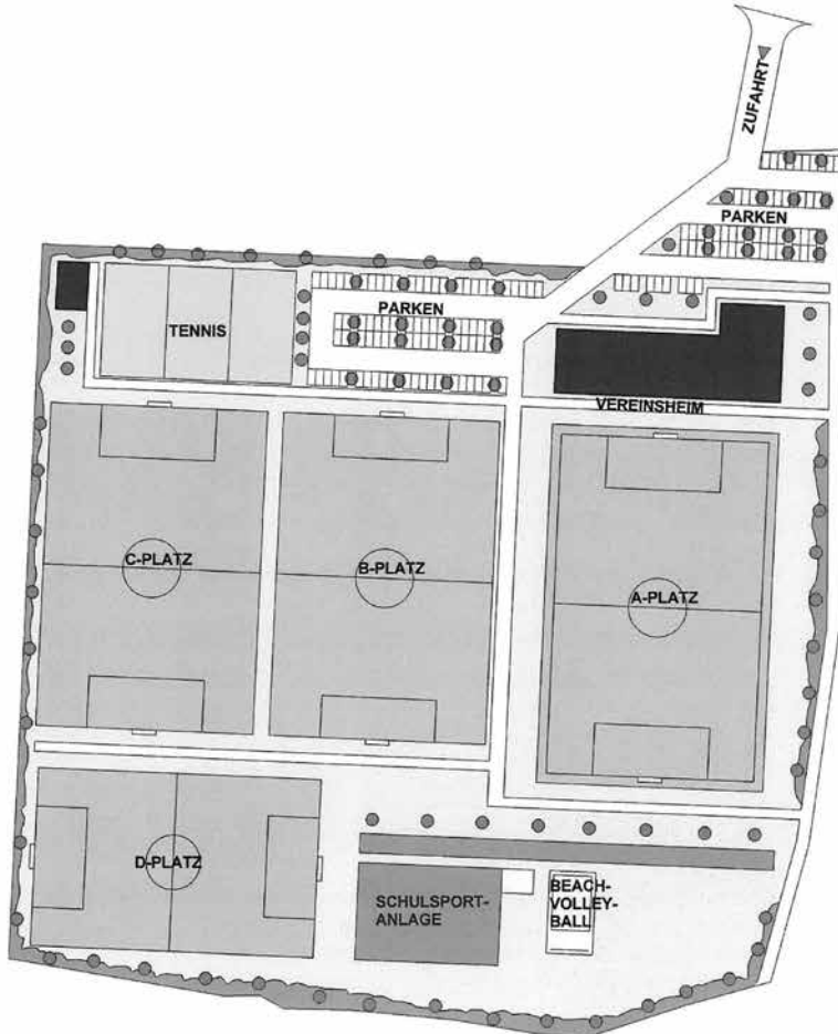
FSV ERLANGEN-BRUCK LAGEPLAN 1:1000
